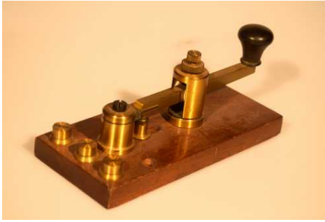
K011 Manipulateur morse Dulci Co London VENDU
